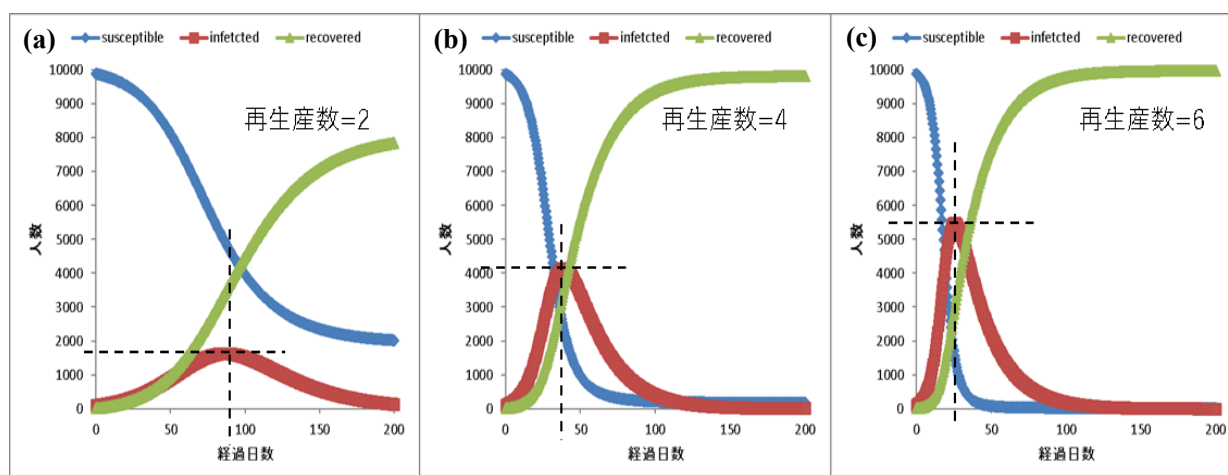
図2 SIRモデルによる数値計算結果. 考慮している集団の人数は10,000人とし, 回復者数の初期値を0人, 初期感染者数を100人, 平均回復期間は20日にそれぞれ固定した上で, 再生産数を(a) 2 / (b) 4 / (c) 6 とした.
