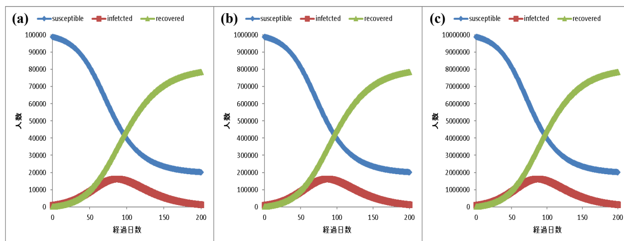
図3 SIRモデルによる数値計算結果. 回復者数の初期値を0人, 再生産数を2, 初期感染者数を100人, 平均回復期間は20日にそれぞれ固定した上で, 考慮している集団の大きさ及び初期感染者数を(a) 100,000人及び1,000人 / (b) 1,000,000人及び10,000人 / (c) 10,000,000人及び100,000人 とした.
