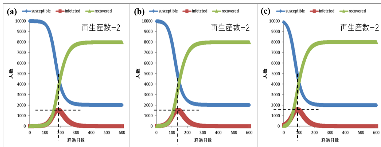
図1 SIRモデルによる数値計算結果。考慮している集団の人数は10,000人とし、回復者数の初期値を0人、再生産数を2、平均回復期間を20日にそれぞれ固定した上で、初期感染者数を(a)1人／(b)10人／(c)100人とした。
