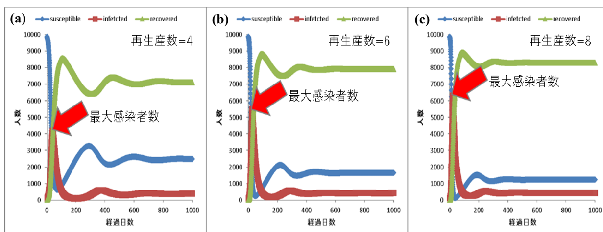
図5 SIRモデルによる数値計算結果。考慮している集団の人数は10,000人とし、感染者数の初期値を100人、回復者数の初期値を0人、平均回復期間を20日、回復者→未感染者に戻るまでの期間を100日にそれぞれ固定した上で、再生産数を(a) 4 / (b) 6 / (c) 8とした。
