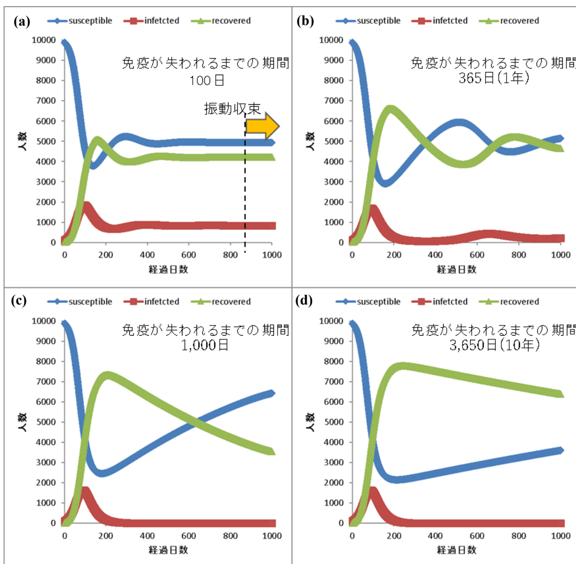
図4 SIRSモデルによる数値計算結果。考慮している集団の人数は10,000人とし、感染者数の初期値を100人、回復者数の初期値を0人、再生産数を2、平均回復期間を20日にそれぞれ固定した上で、回復者→未感染者に戻るまでの期間を(a) 100日 / (b) 365日 / (c) 1,000日 / (d) 3,650日とした。
